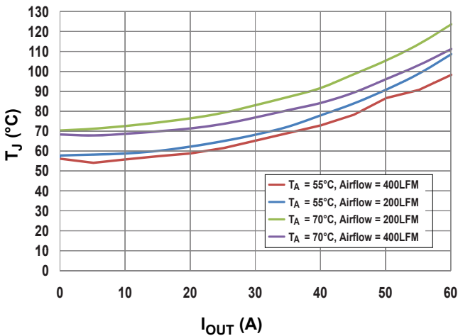
Thermal Evaluation
