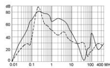
450A (FMAC-0957-H550)
