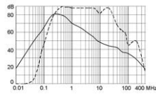
25A (FMAC-0932-2510L)
