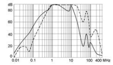
36A (FMAC-0934-3610)
