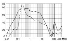
340A (FMAC-0956-H410)
