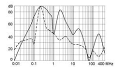
550A (FMAC-0957-H650)
