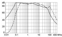
36A (FMAC-0932-3610L)
